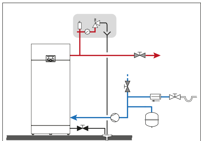
Fig. 27. Llenado típico del sistema
