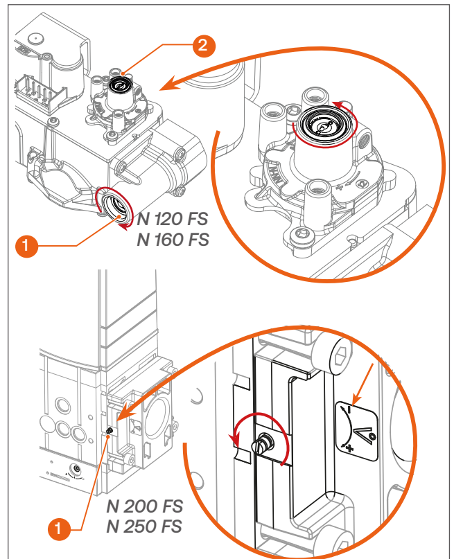
Fig. 19. Ajuste previo del tornillo de caudal de gas para propano
