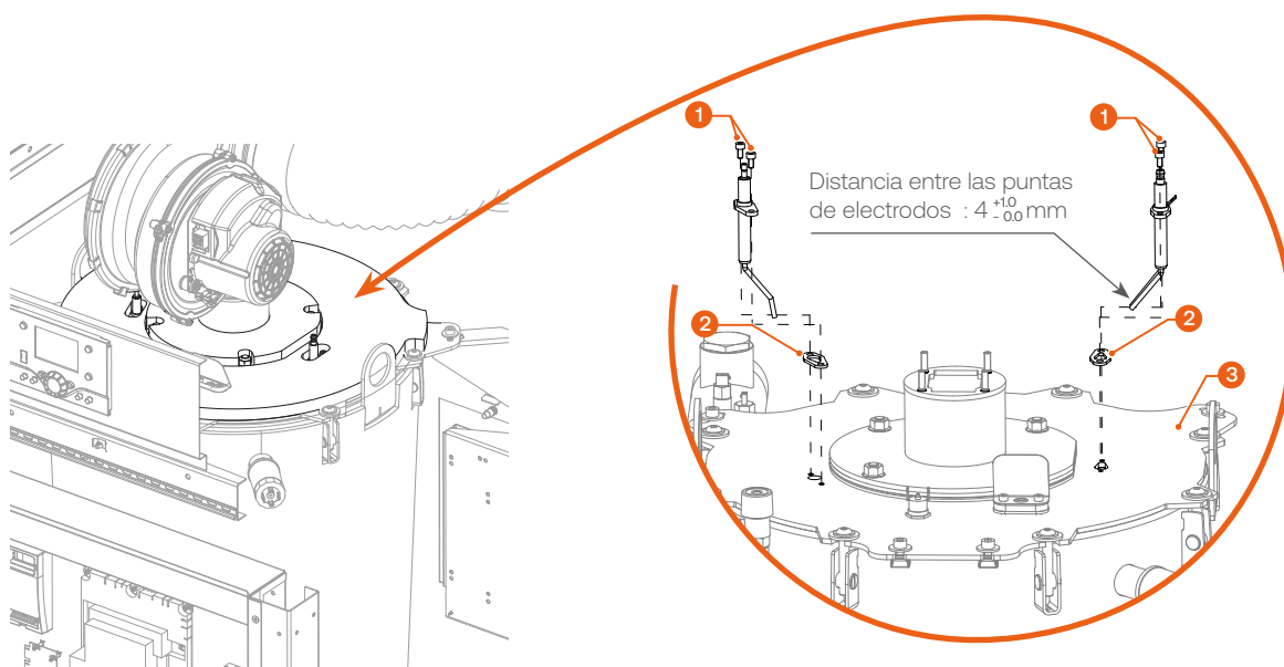
Fig. 30. Extracción e instalación de los electrodos
