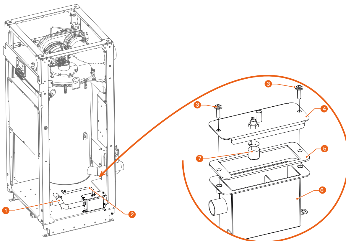
Fig. 29. Limpieza del conducto de condensados y el sifón
