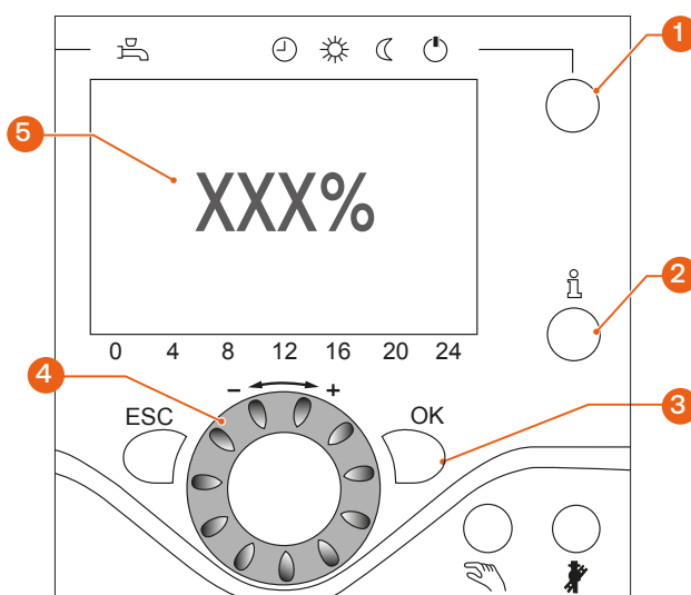
Fig. 21. Ajuste de la combustión - panel de control
